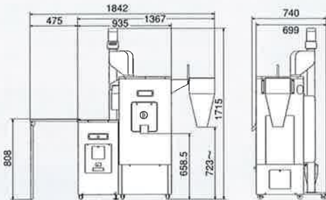
石抜付精米機 SR2231ESC (コインタイマー仕様)
