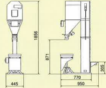
白米計量機 IK150H
