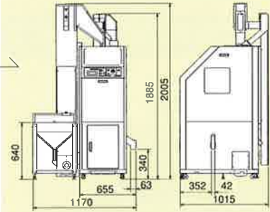
色彩選別機 CLX352DF-S
