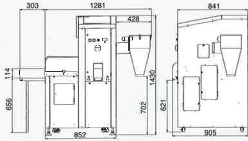
石抜付精米機 SR3740RD SR3740RS (コインタイマー仕様)
