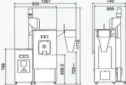
石抜付精米機 SR2230ES
